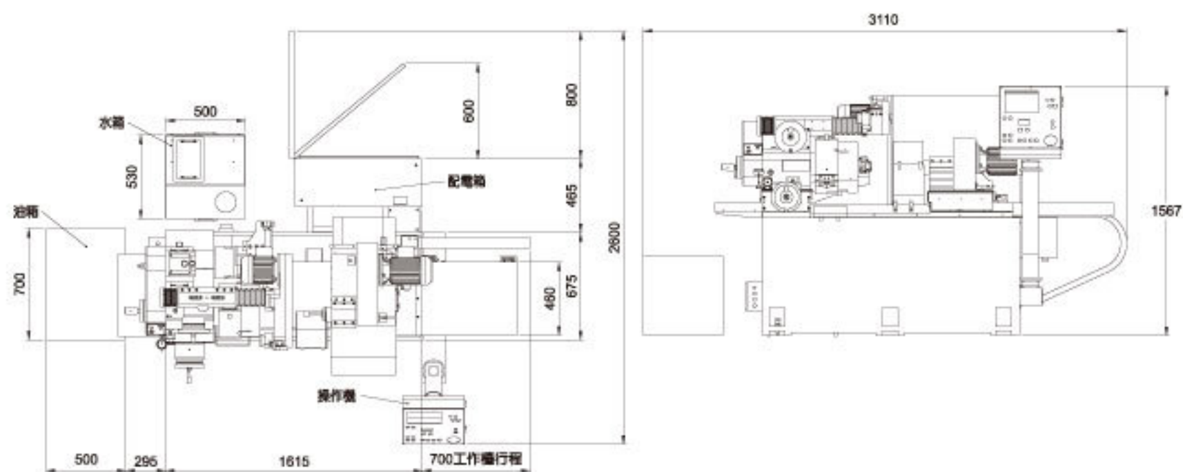
機器尺寸圖 JHI-150NC
