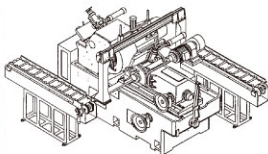
JHC-2412 CNC 4 型無心磨床及 機械手自動送料、收料系統
