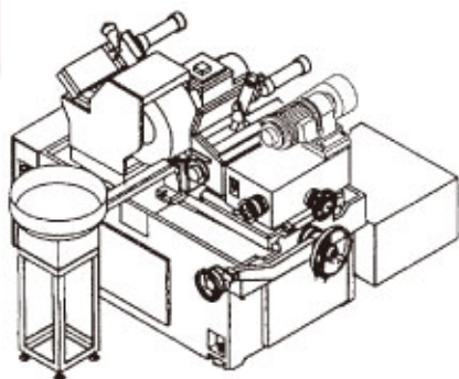
JHC-18 型無心磨床及振動送料
