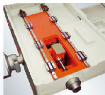
JHC-24H型下滑台之設計
