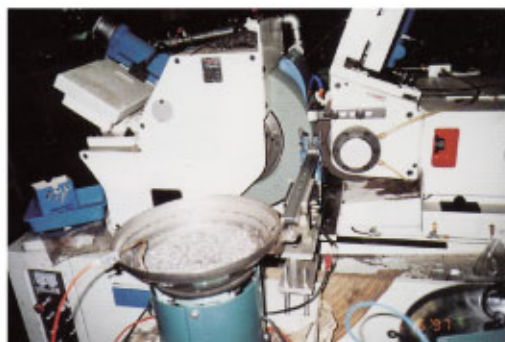
JHC-18 型無心磨床及振動送料
