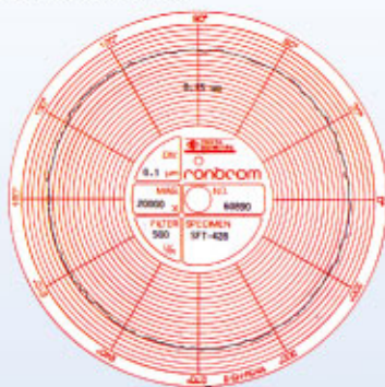
真圓度
